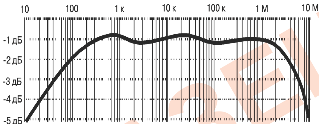
Рис.3 Амплитудно-частотная характеристика
