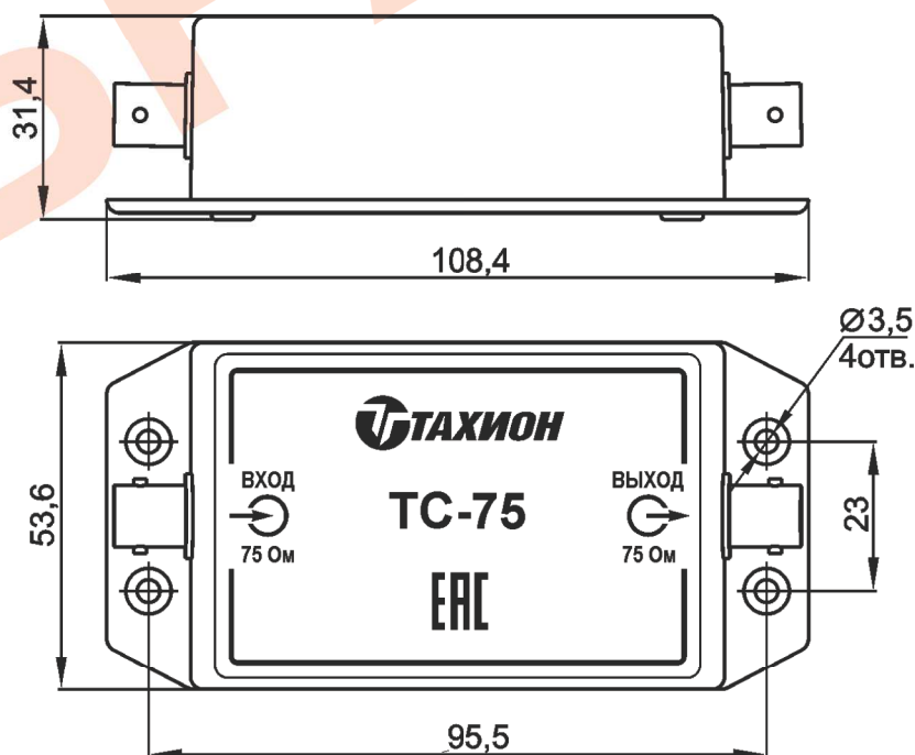
Рис.1 Габаритные и установочные размеры
