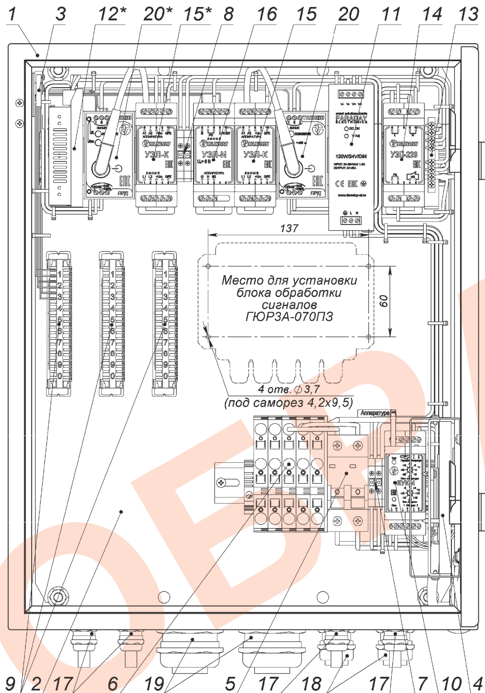
Рис. 2. Устройство термощкафов ТШ-3-05 и ТШ-3-06 (дверь открыта на 90°) * для исполнения ТШ-3-06 отсутствуют
